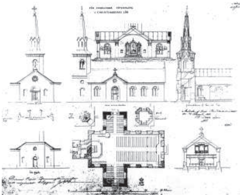
Ritning av nya kyrkan
