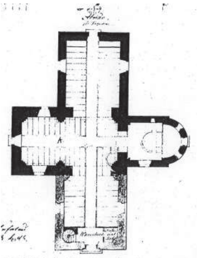
Ritningen över förslaget till utbyggnad av gamla kyrkan
